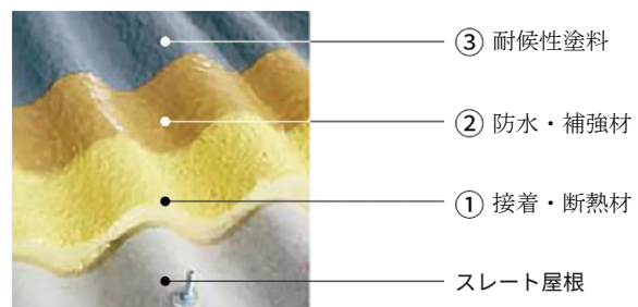
<SOSEI 工法：3層特殊樹脂構造>
